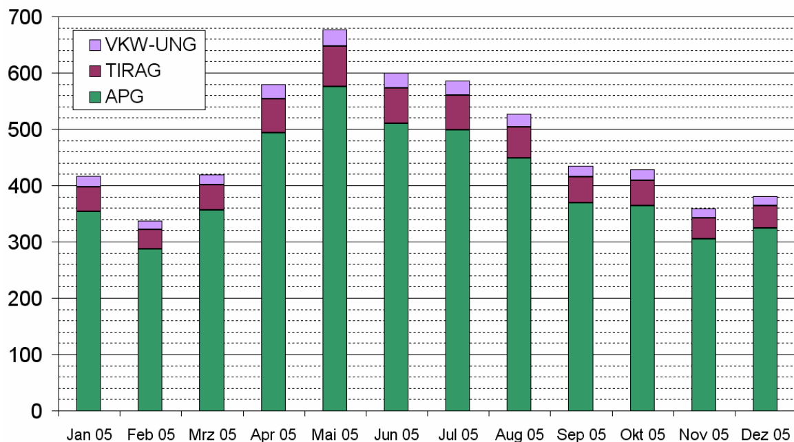
Monatlich zugewiesene Ökostrommengen in GWh
